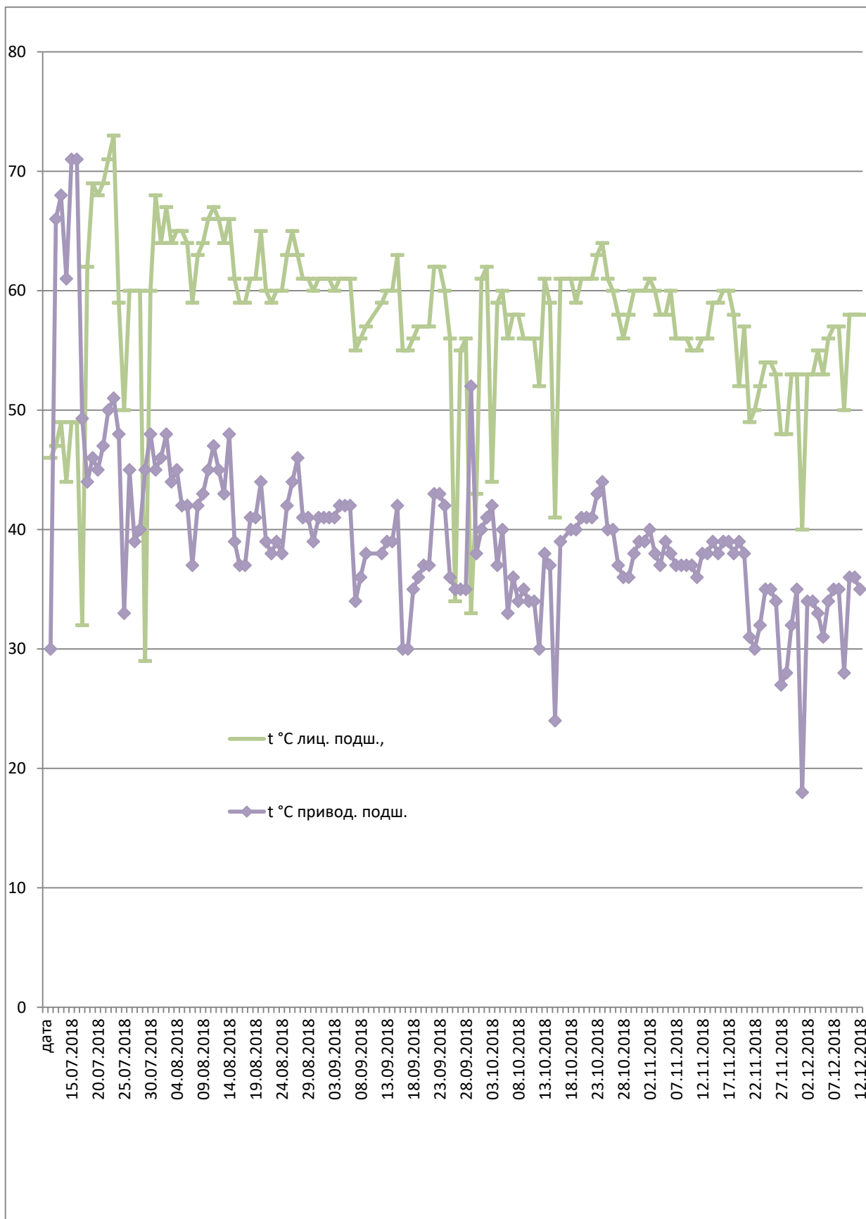
Электродвигатель воздуходувки №3:
